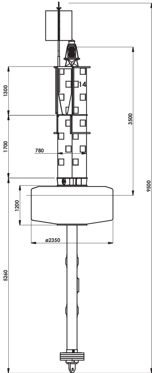
EBM-HV 24 de 2,35m de diámetro.
